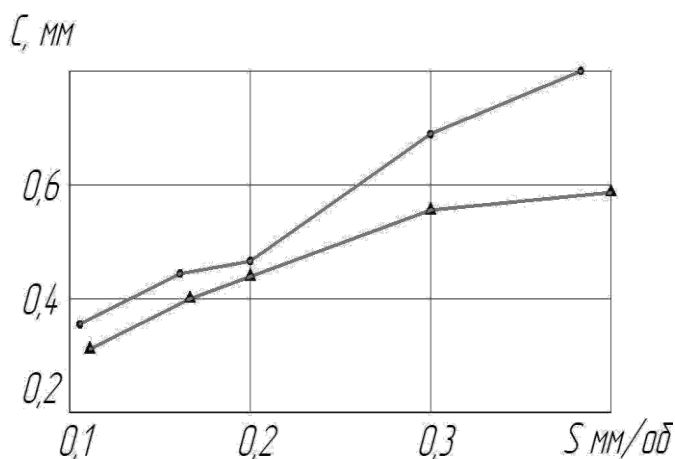
2 - сурет – Контакт ауданының жіберуге тәуелділігі
