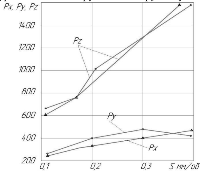
3 - сурет – Жоңқа отыруының жіберуге тәуелділігі
