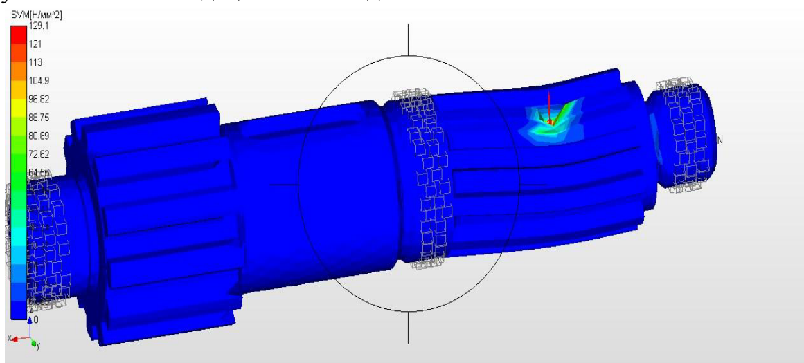
18 – сурет - Оймакілтекті қосылыс тісіндегі кернеу
