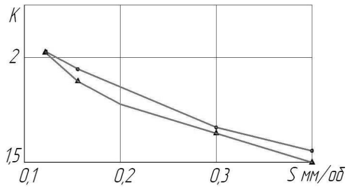
3 - сурет – Жоңқа отыруының жіберуге тәуелділігі
